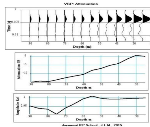
PSV : Atténuation (Document IFP School)
