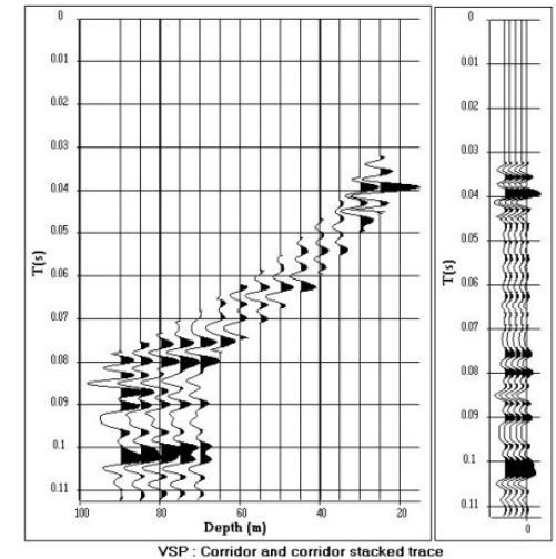
PSV : Trace sommée dans un couloir de sommation (Document IFP School)
